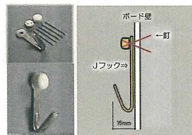
石膏ボード用フック(例)
